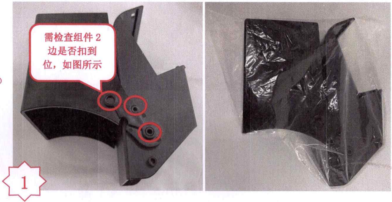
图一, 检查 PA2417 是否装配到位, PA2417 是带有 PE 袋的
